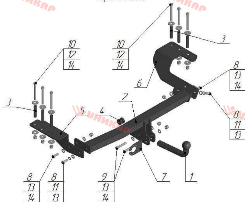
Тягово-сцепное устройство Haval H6 (Арт. 10121А)
